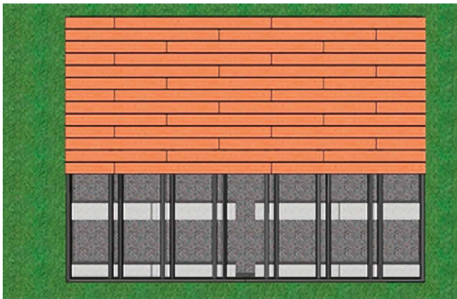
Unterbau, UK und Deck bei 1/3 Längensversatz. Achismaße: 500-117-500-117-500 mm
