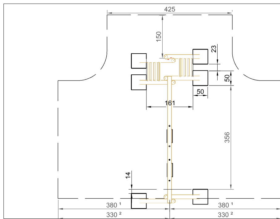
Sicherheitsbereich und Fundamentplan
